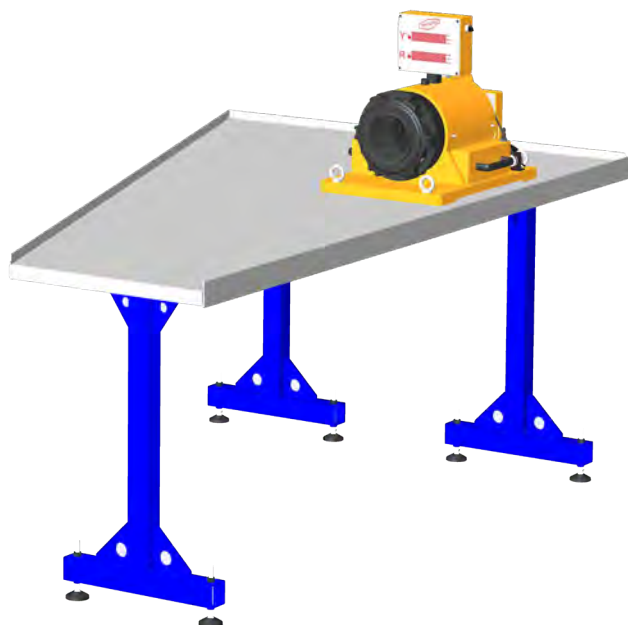
■ Art. A100/P Posizionatore a 2 assi x TB80, TB100, TB130 Two-axis positioner x TB80, TB100, TB130
