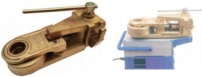
Art. 087 - Morsa su Medibender MD070 e MD083 per imbutire, flangiare, calibrare tubi. Art. 087 - Vice accessory on Medibender MD070 e MD083 for chamfering, flanging, calibrating tubes.
